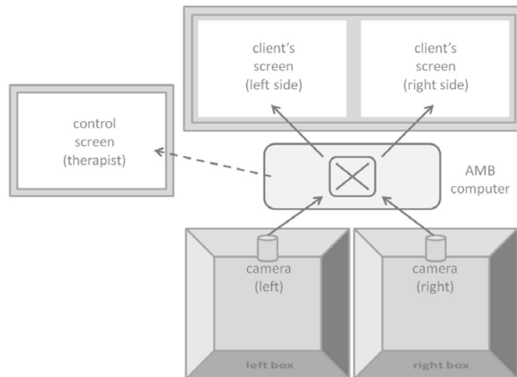
Figure 2: Schematic Overview of AMB setup
